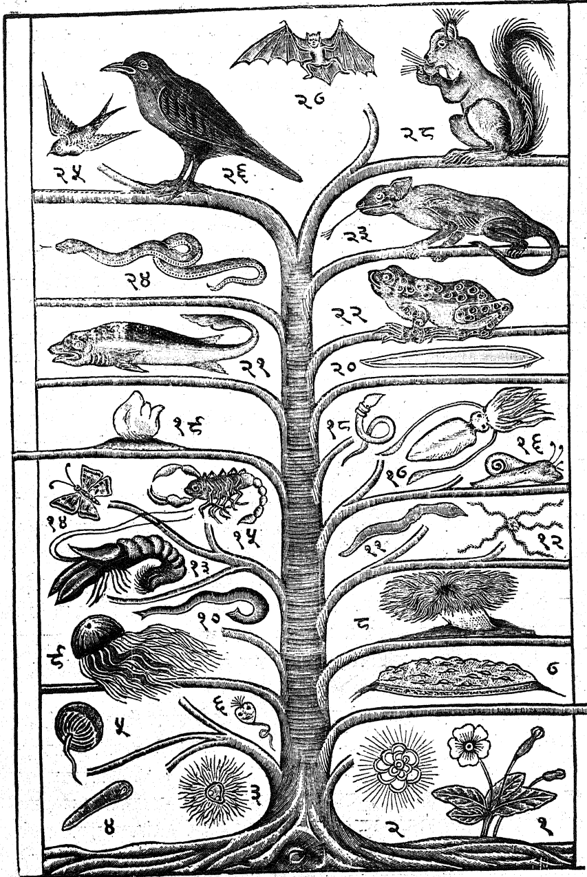
चित्र ६६—चर प्राणियों का वंश-वृत्त ।
